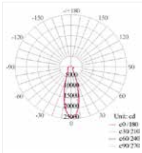
30° Óptica
