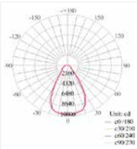
60° Óptica
