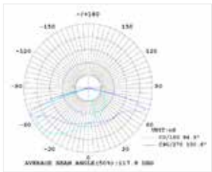
140°x100° Óptica
