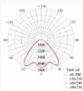
90° Óptica
