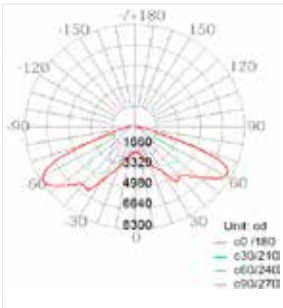
80°x150° Óptica
