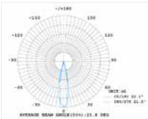
20° Óptica
