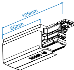
Alimentación carril JA110
