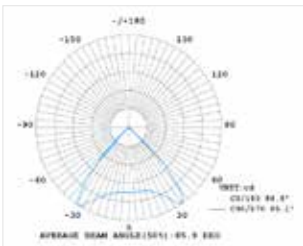
90° Óptica
