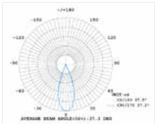
40° Óptica
